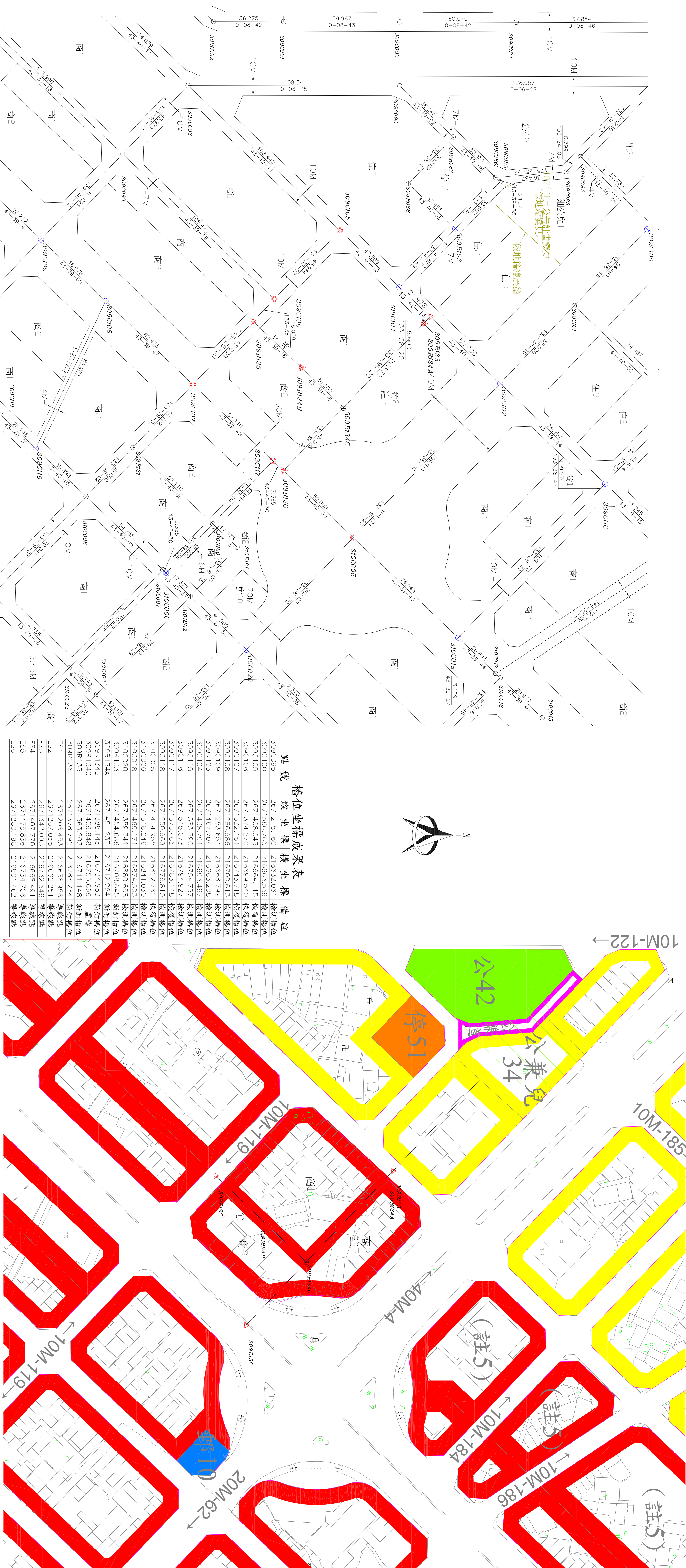
都市計畫樁位公告圖 SCALE=1/1000
