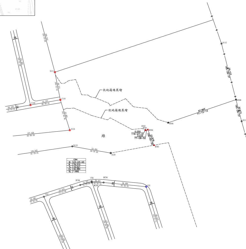
變更後都市計畫樁位圖 SCALE=1/1000
