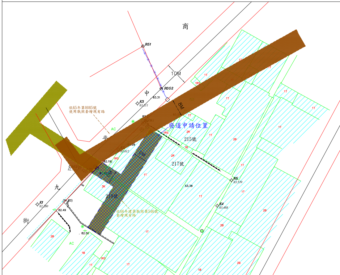
現況圖 S=1:500
