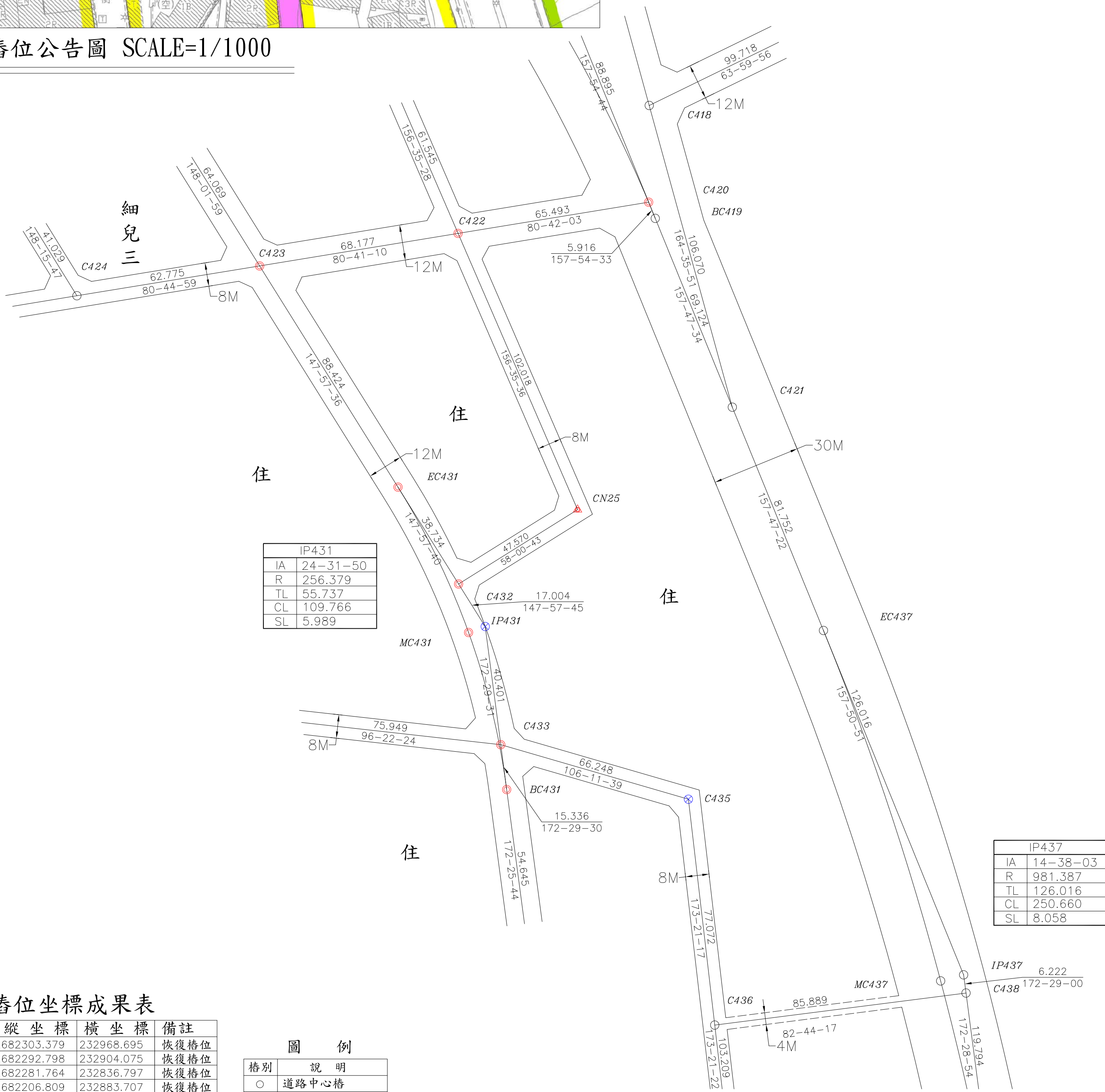
修正後樁位圖 SCALE=1/1000
