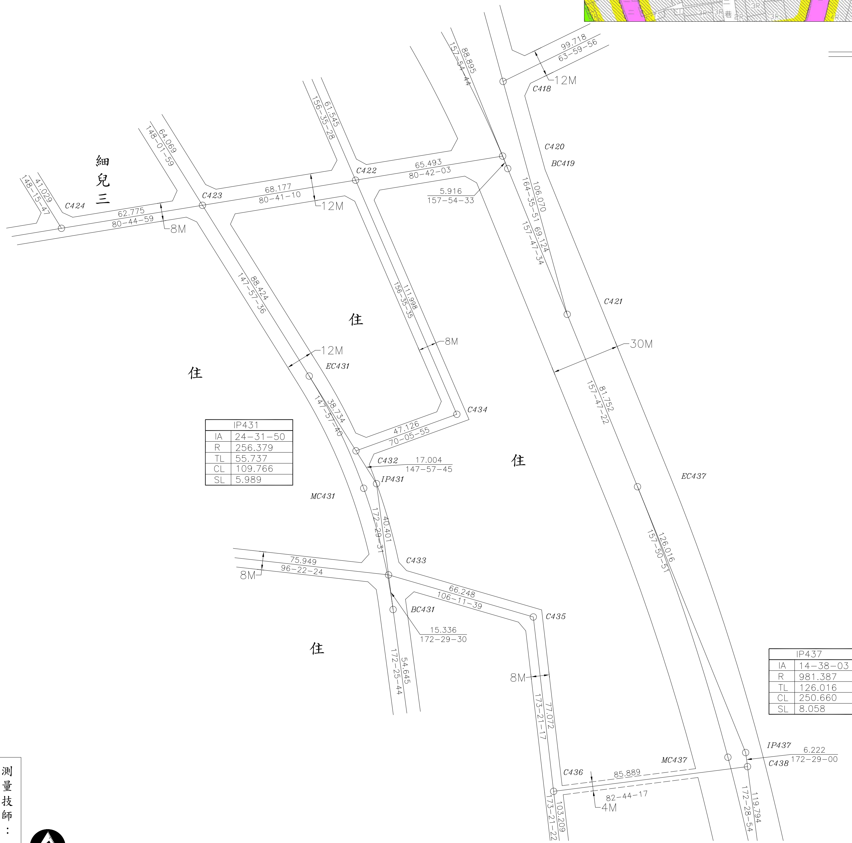
都市計畫樁位公告圖 SCALE=1/1000
