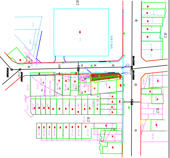
地籍套繪圖 S=1:600
