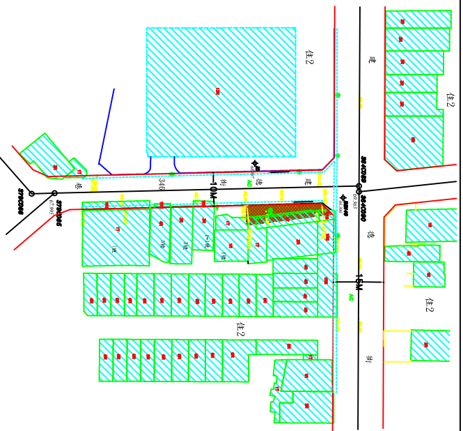
現況圖 S=1:600
