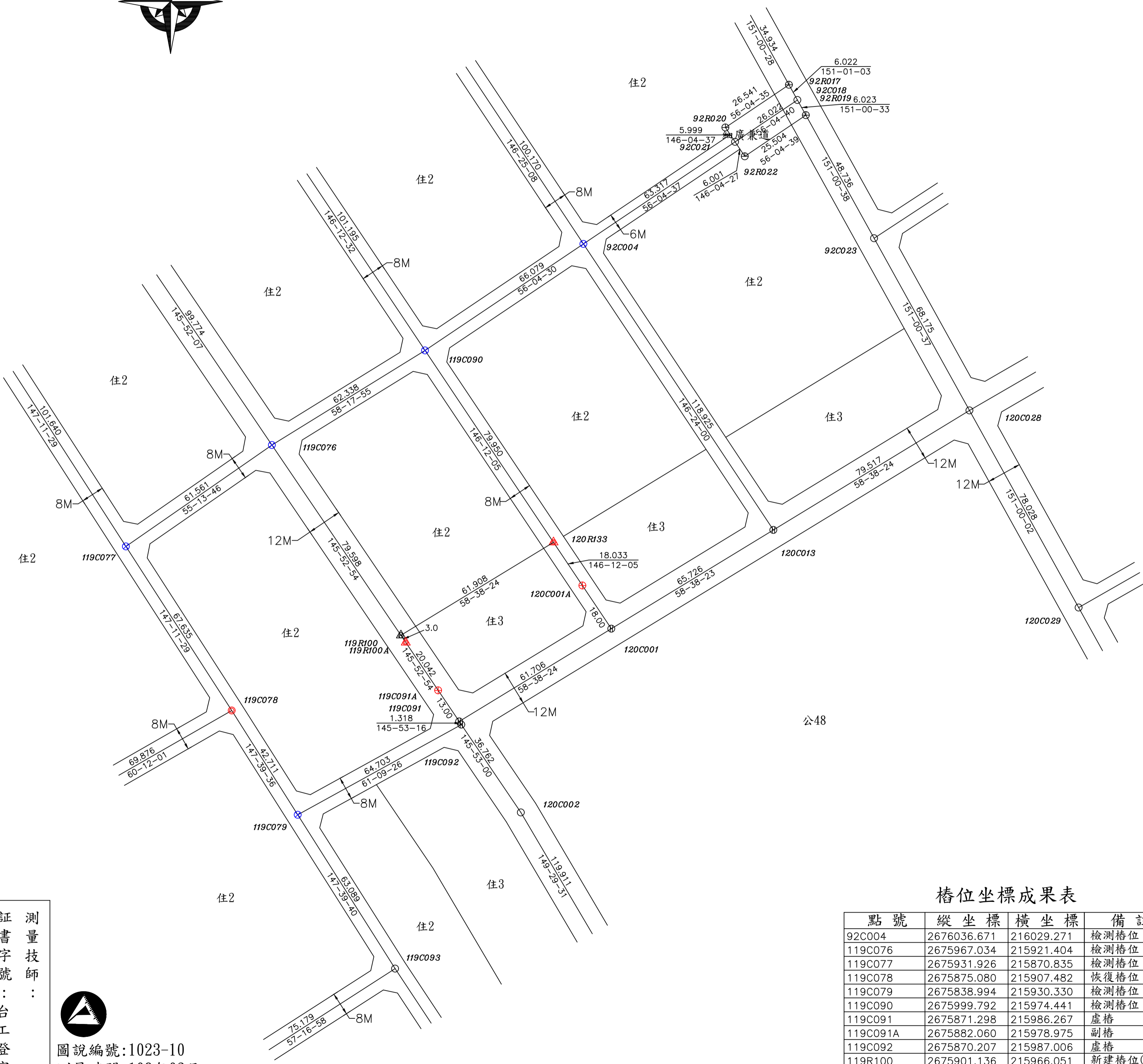
樁位圖 SCALE=1/1000
