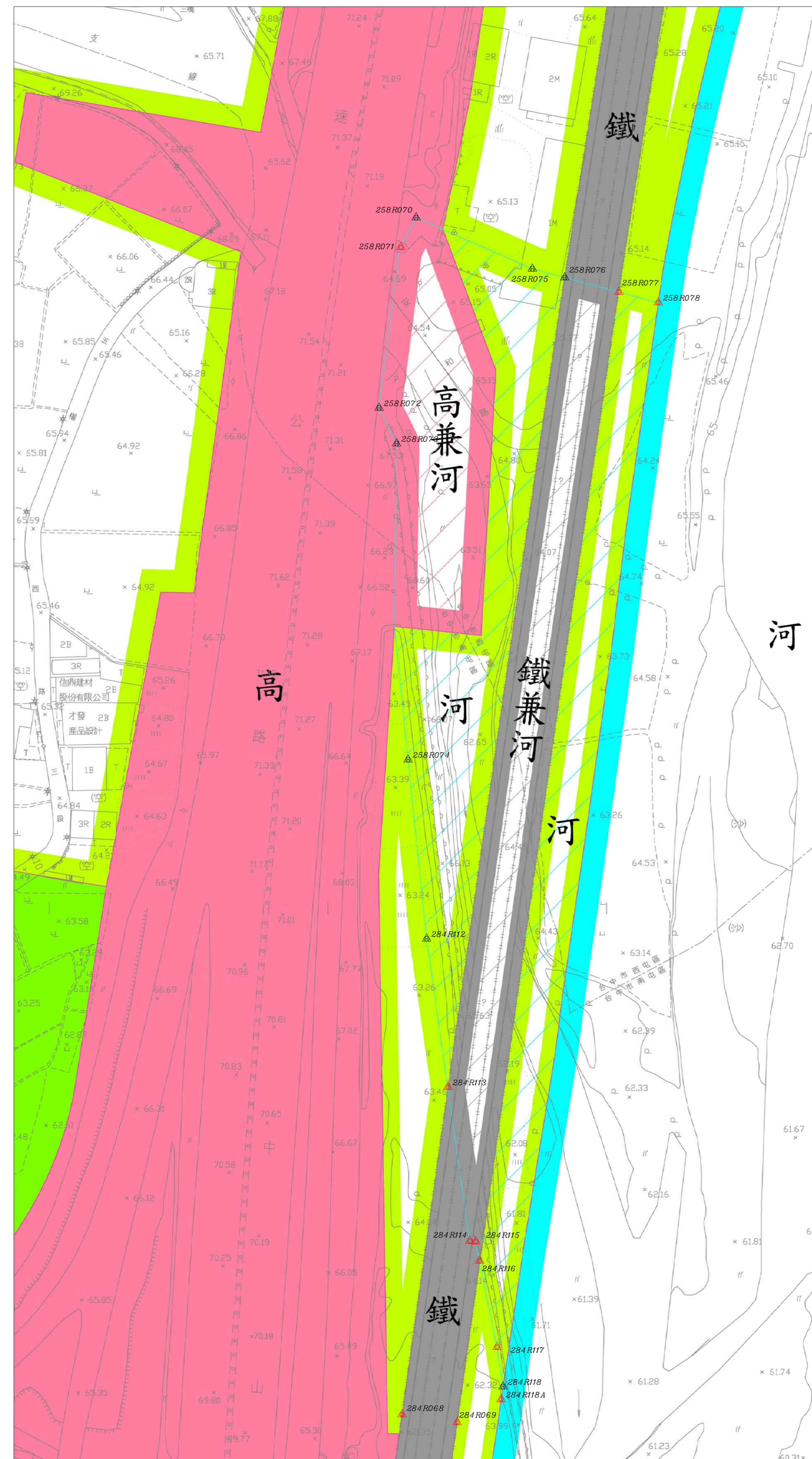
都市計畫橋位公告圖 SCALE=1/1000
