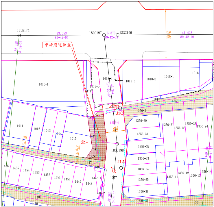
地籍套繪圖 S=1/500
