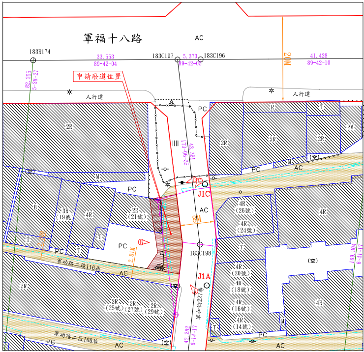
現況圖 S=1/500
