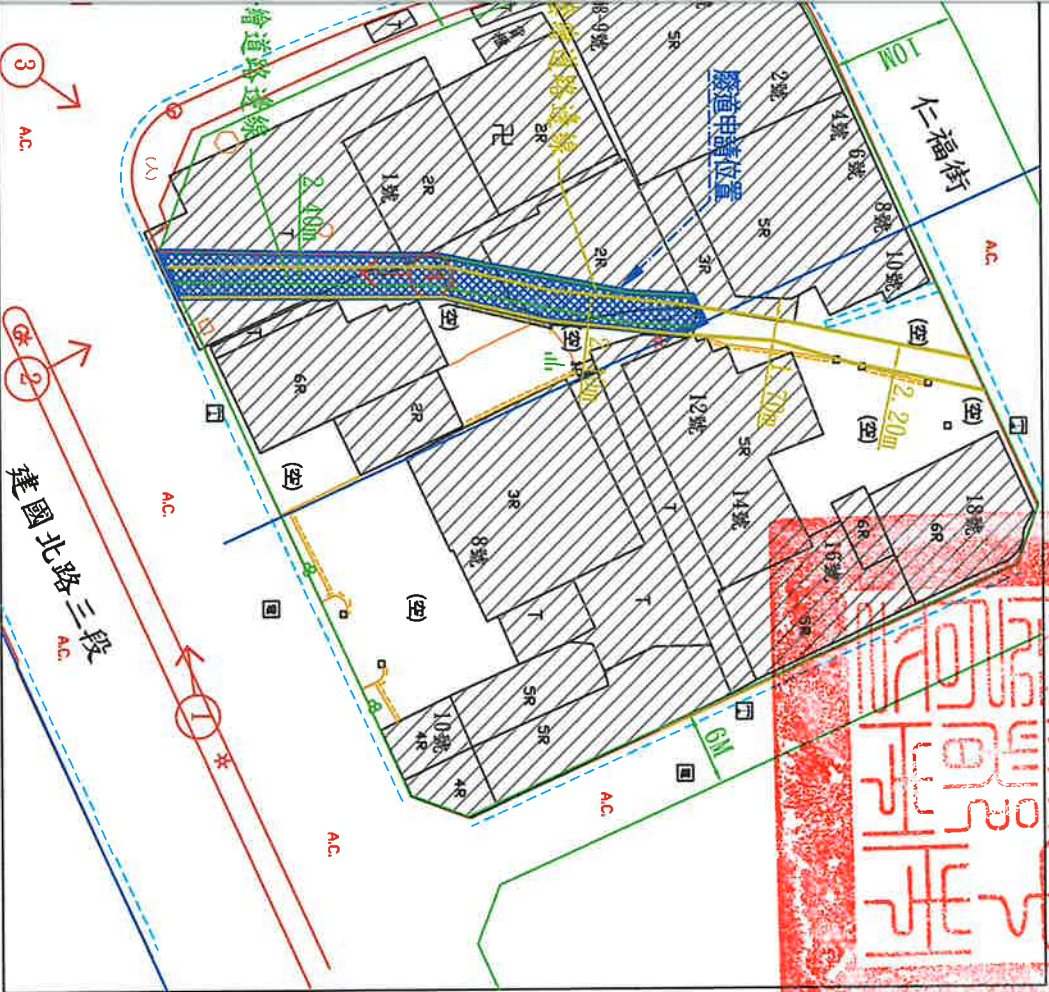
現況圖 S=1:600
