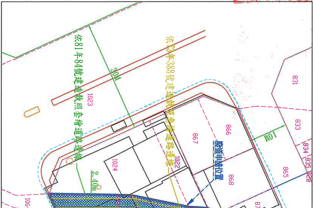
地籍套繪圖
