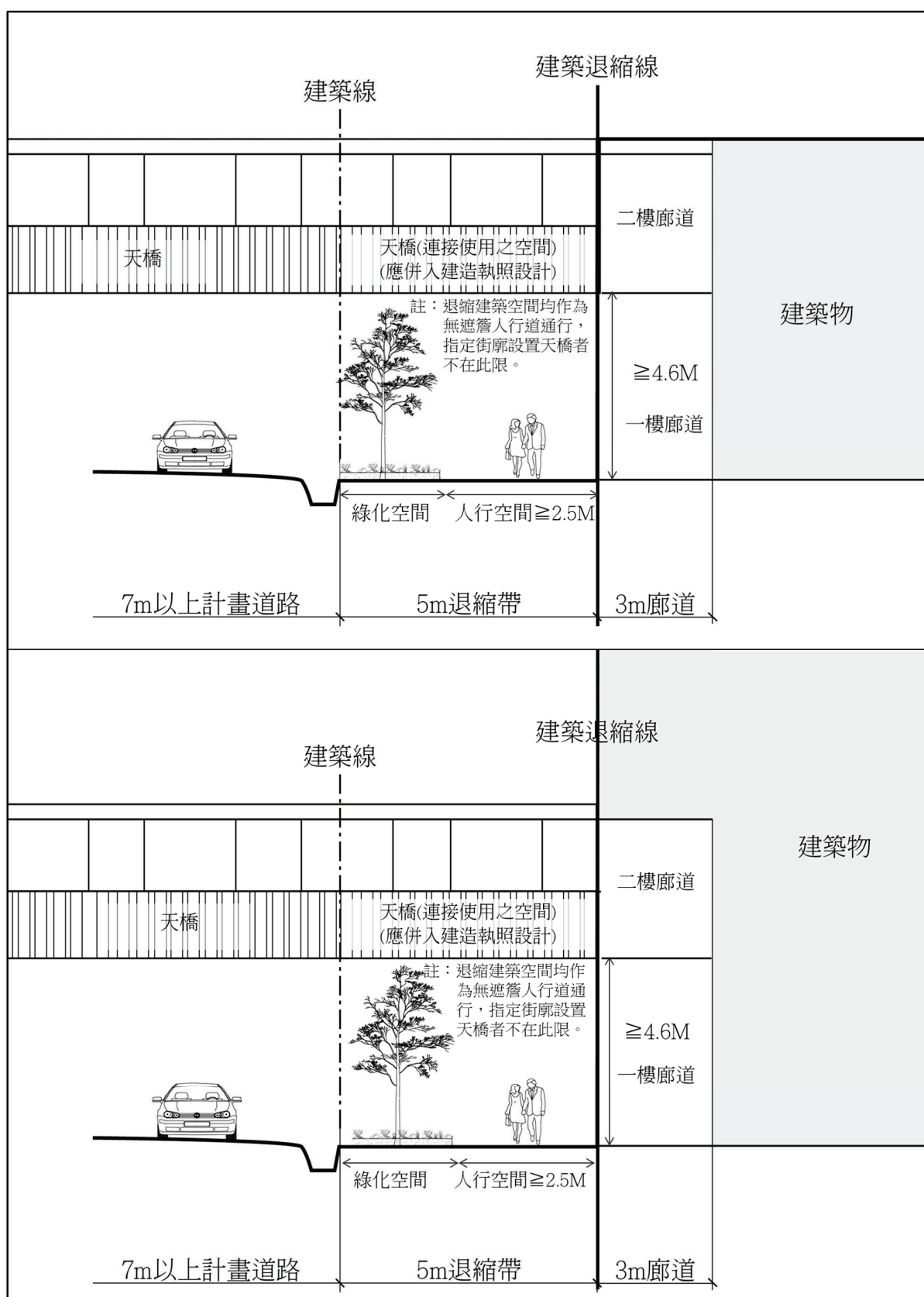
圖 6 臨接臨 7 公尺（含 7 公尺）以上計畫道路退縮空間斷面參考示意圖
