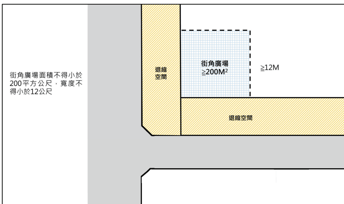
圖 7 指定街角廣場劃設參考示意圖
