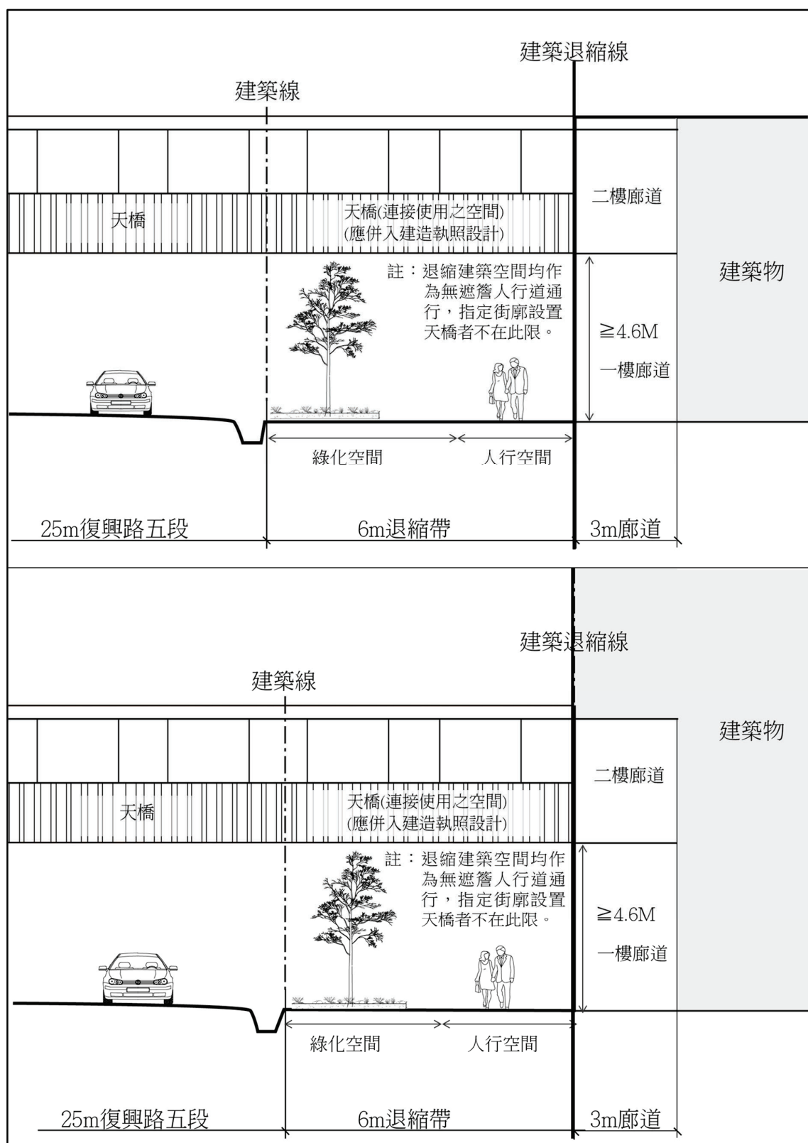
圖 4 臨接復興路五段退縮空間斷面參考示意圖
