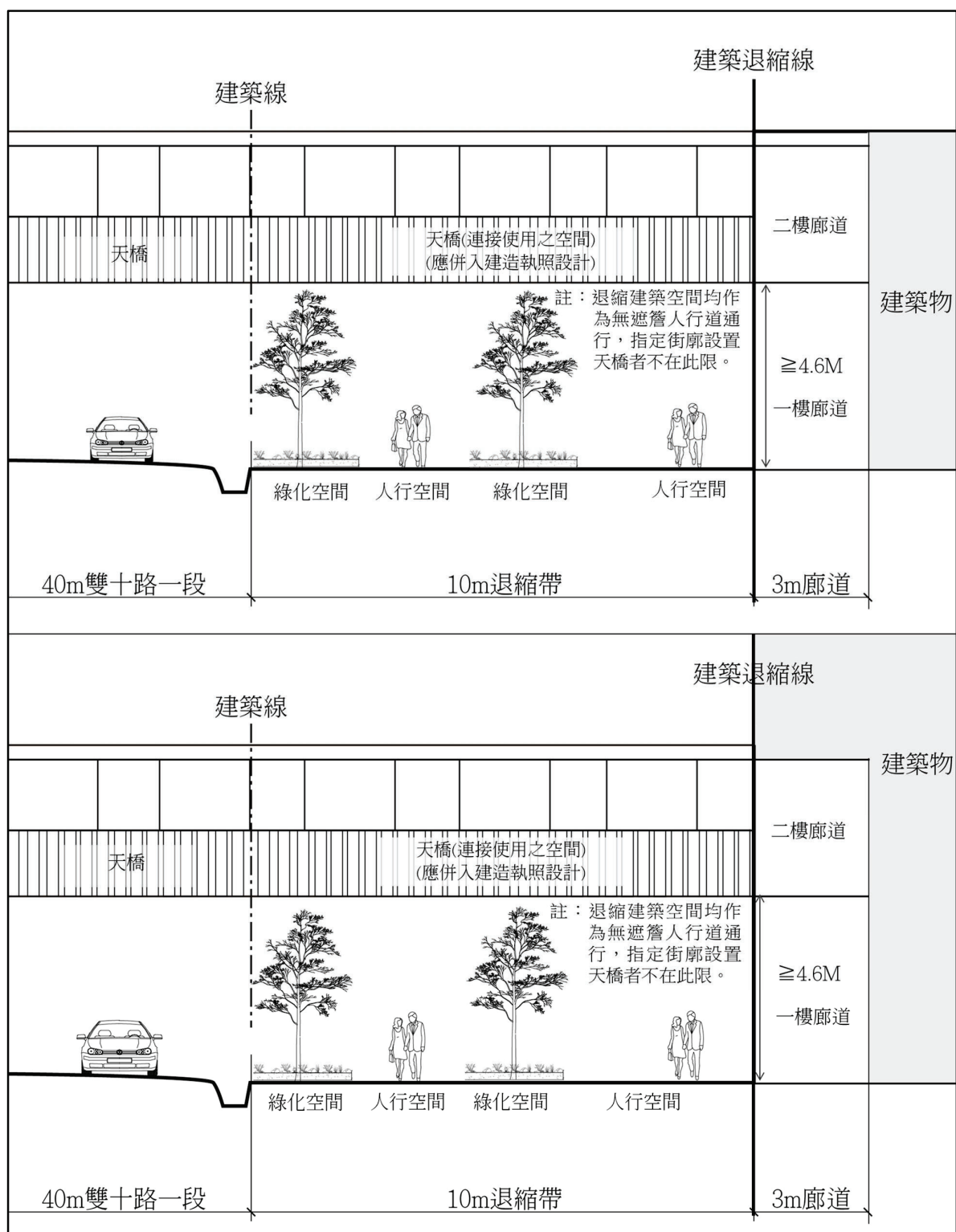
圖 5 車站用地臨雙十路一段退縮空間斷面參考示意圖
