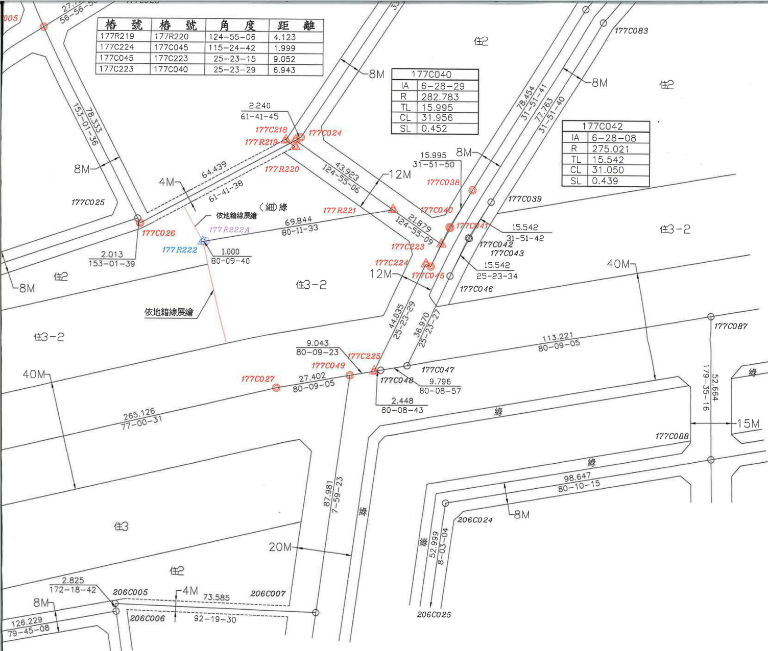
變更後樁位圖
