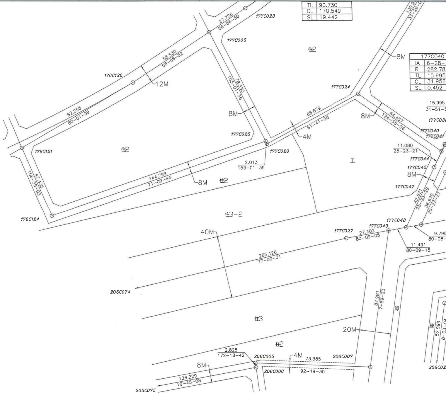
變更前樁位圖
