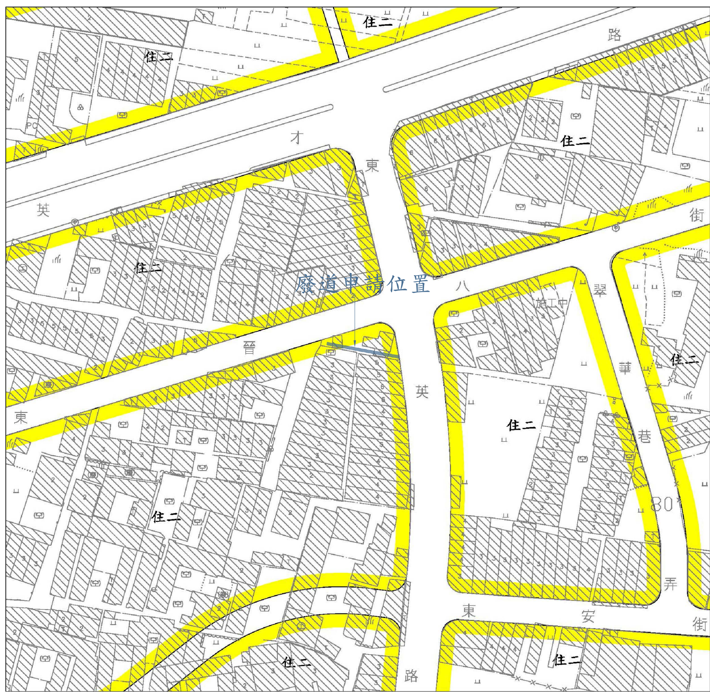
都市計畫圖 S=1:1000
