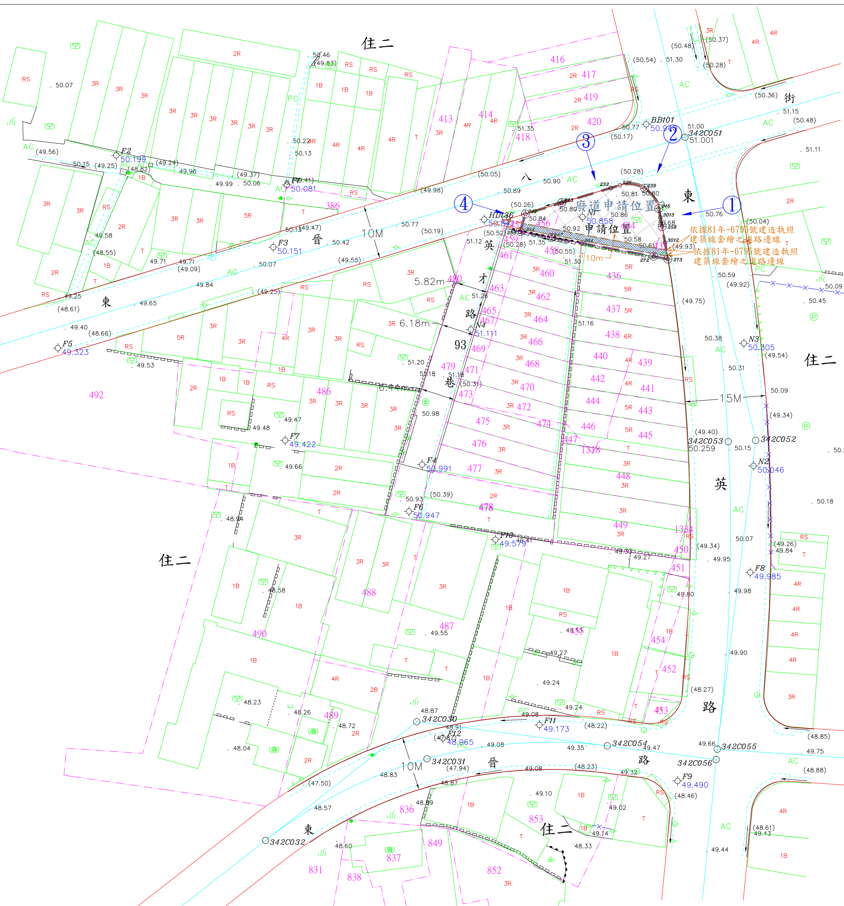
地籍套繪圖 S=1:500
