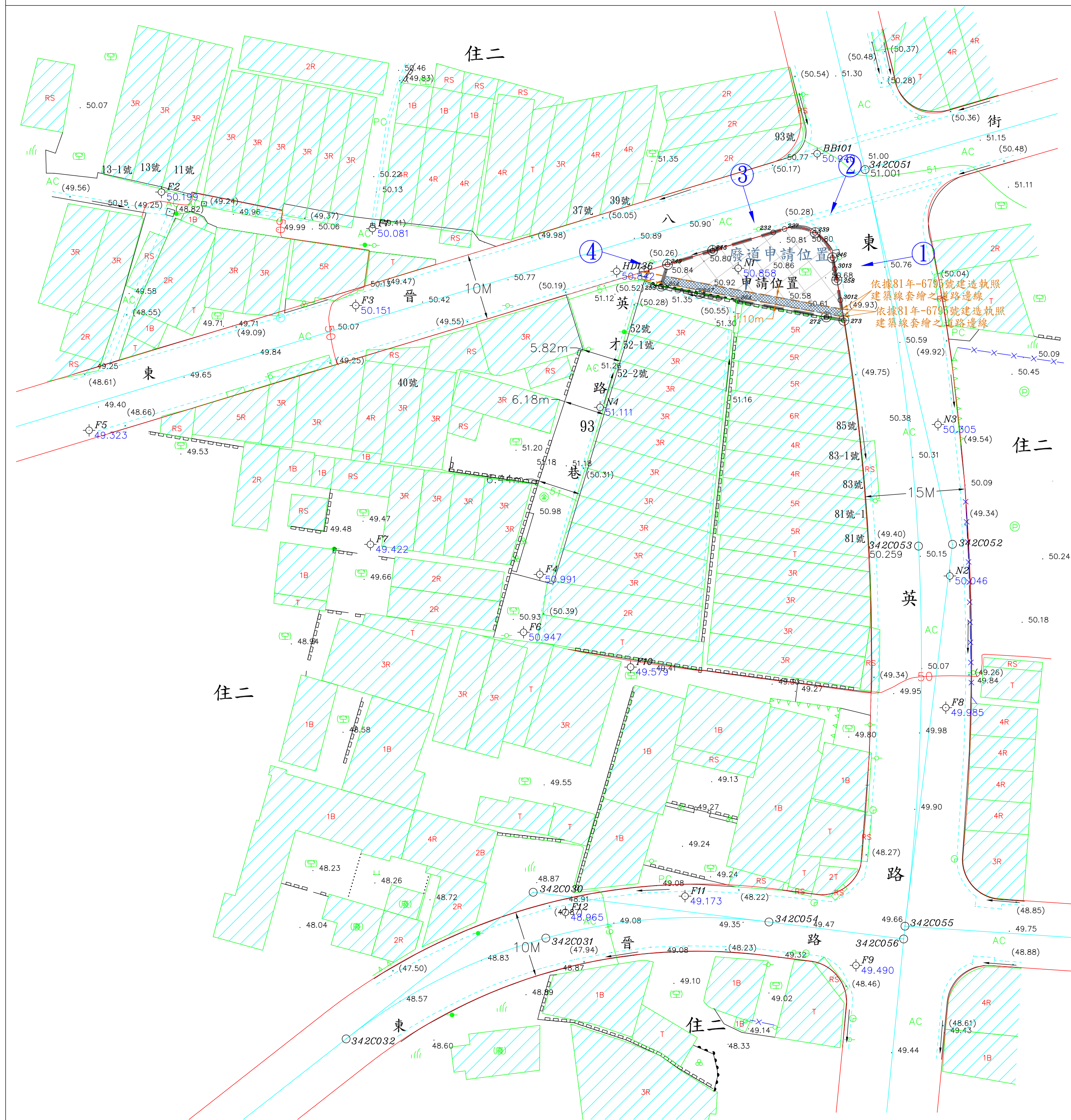
現況成果圖 S=1:500
