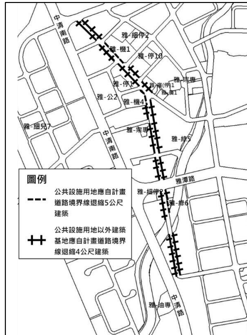
大雅都市計畫指定路段建築基地退縮規定示意圖
