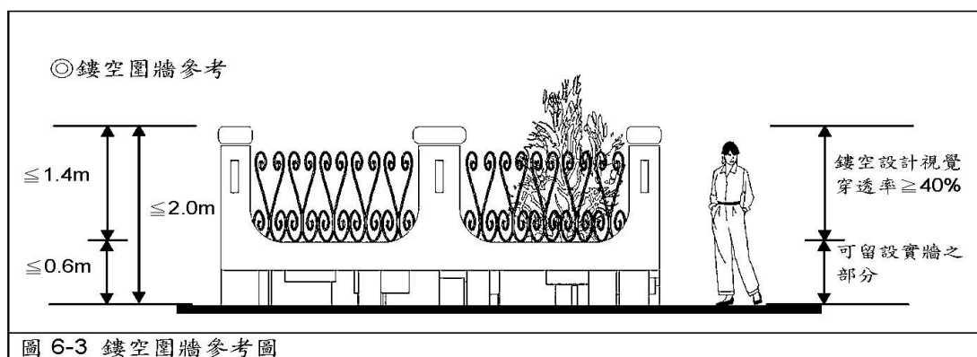
圖 6-3、住宅區建築物前院鑲空圍牆示意圖
