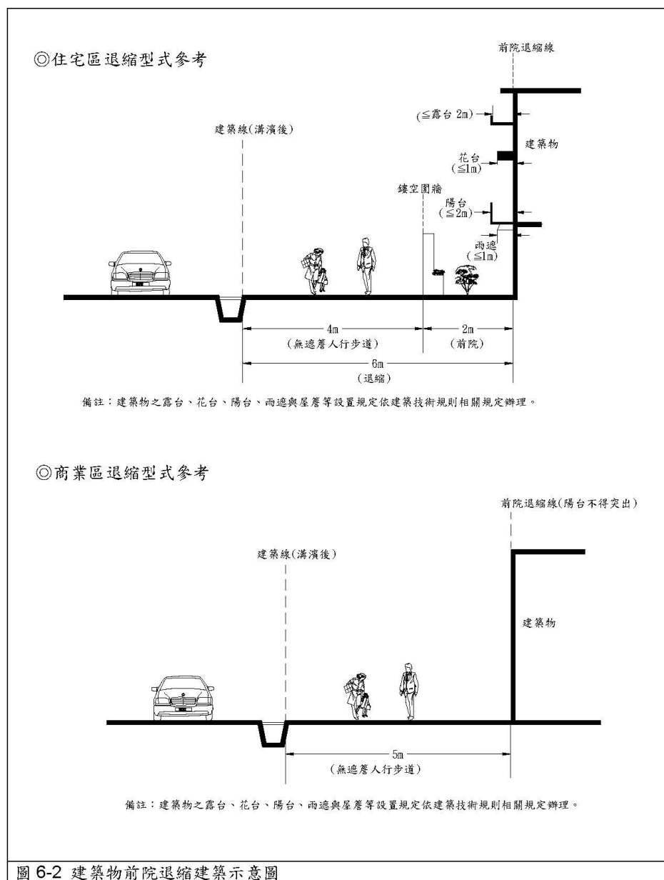
圖 6-2、住宅區建築物前院退縮建築示意圖
