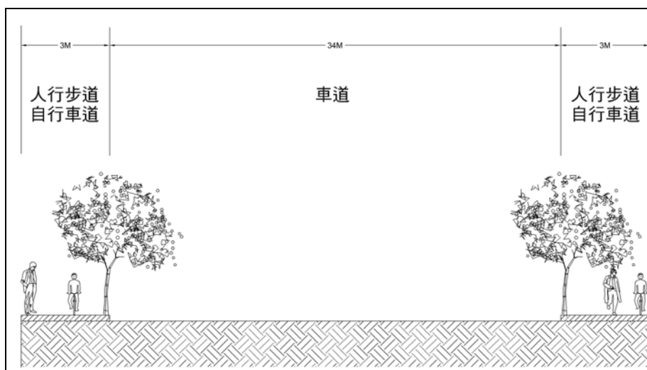
附圖十 40M-3 計畫道路斷面設計示意圖
