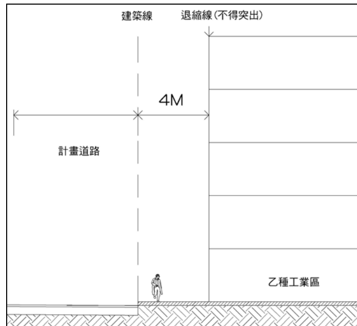
附圖三 工業區建築基地退縮斷面設計示意圖
