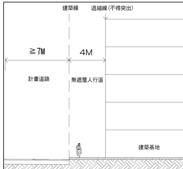
附圖一 住宅區、商業區及市場用地建築基地(選擇)無遮簷人行道退縮斷
