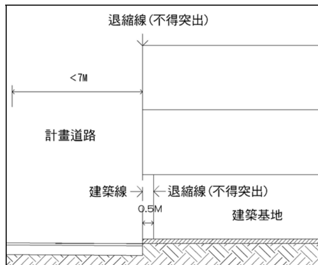
附圖二 住宅區、商業區及市場用地建築基地面臨現有巷道退縮斷面設計
