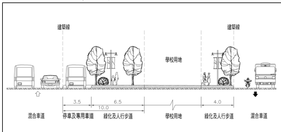
附圖四 文中、文小用地建築基地退縮斷面設計示意圖
