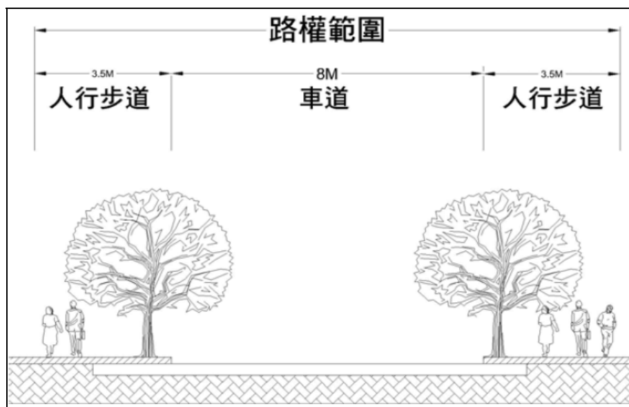
附圖九 細 15m-1 斷面設計示意圖
