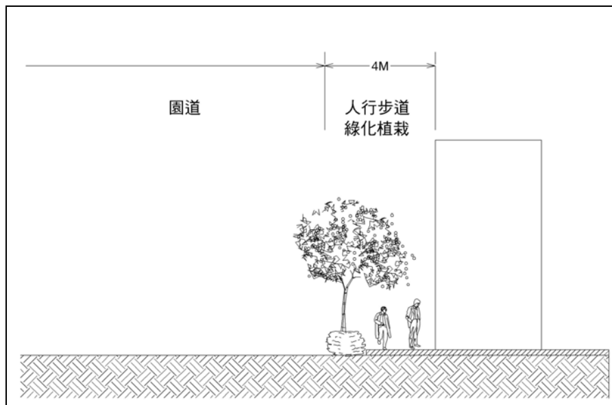
附圖八 園道兩側建築基地退縮斷面設計示意圖
