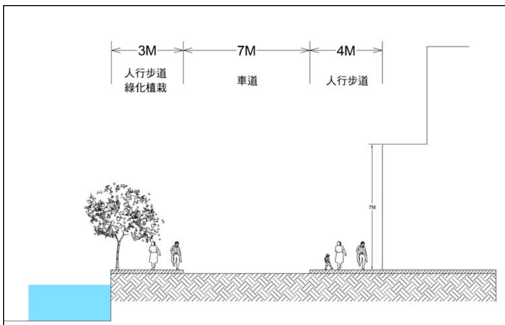
附圖七 排水道用地兩側道路與建築基地退縮斷面設計示意圖
