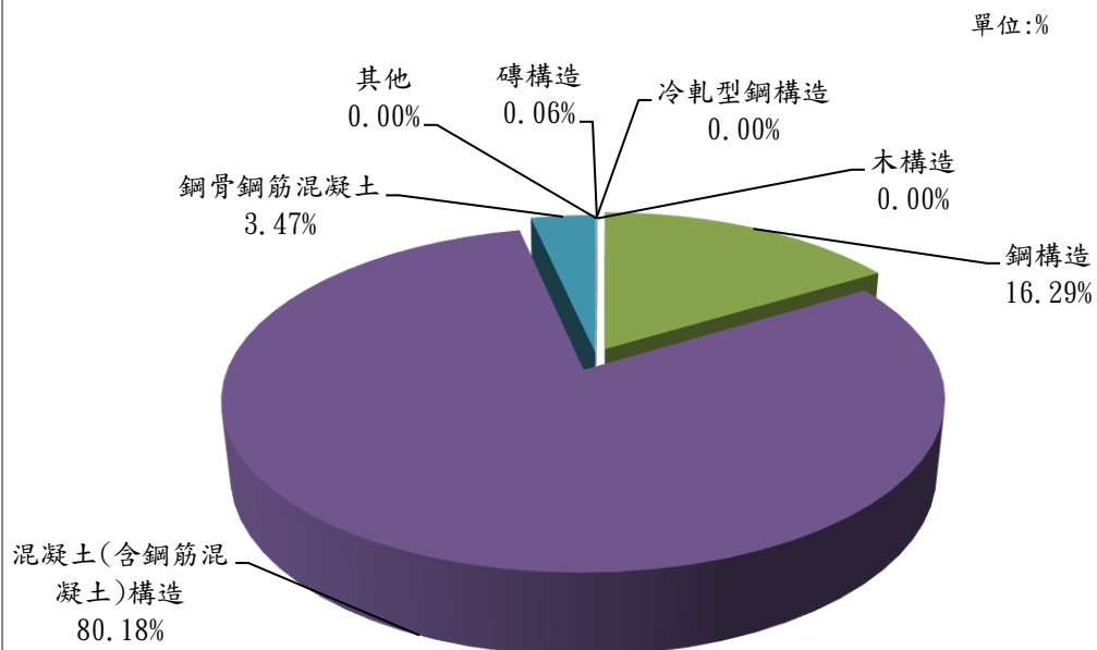
圖10. 106年核發建築物使用執照 總樓地板面積-按構造分
