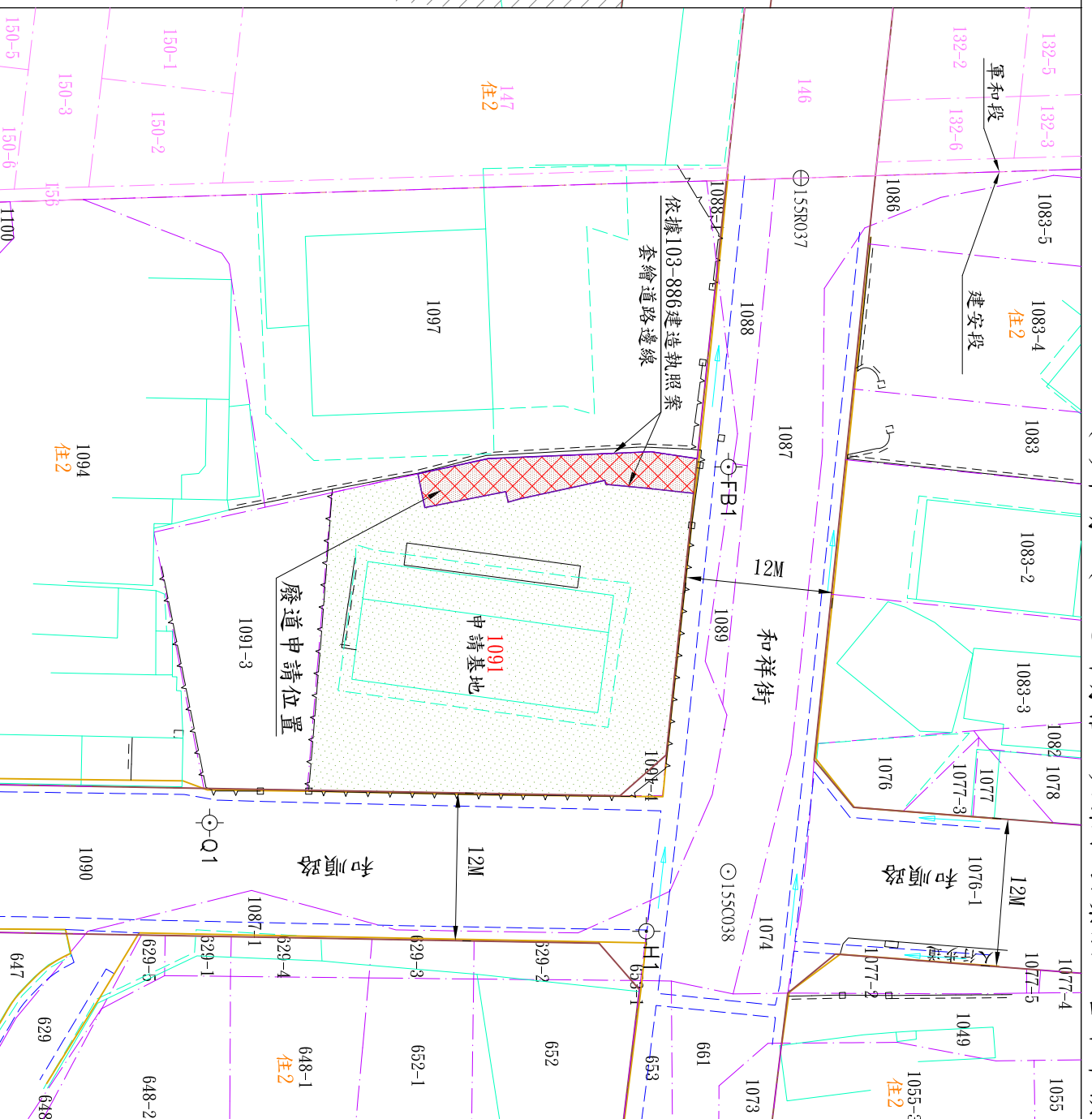
地籍套繪圖 S=1:500
