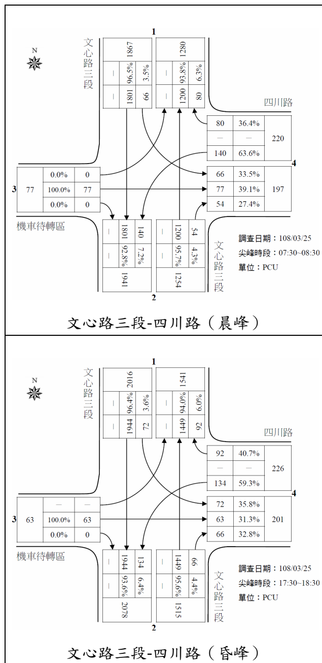
圖 1-2 基地鄰近路口尖峰小時轉向流量示意圖 (續)
