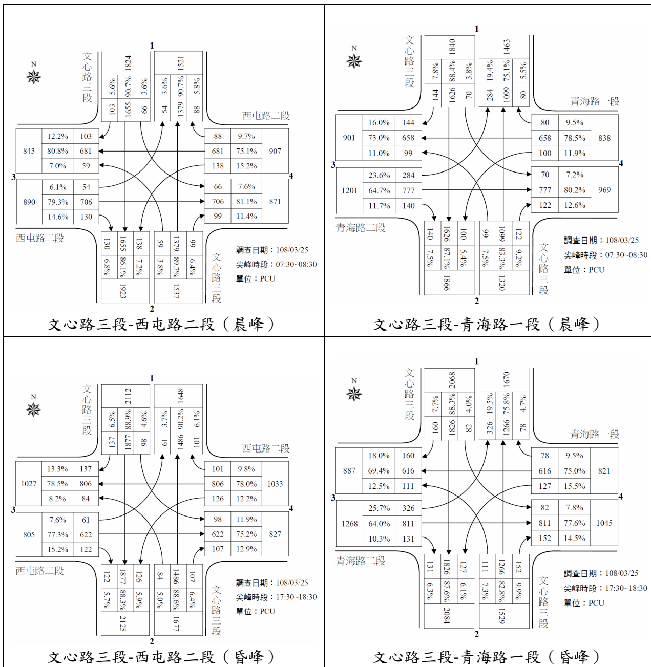
圖 1-2 基地鄰近路口尖峰小時轉向流量示意圖
