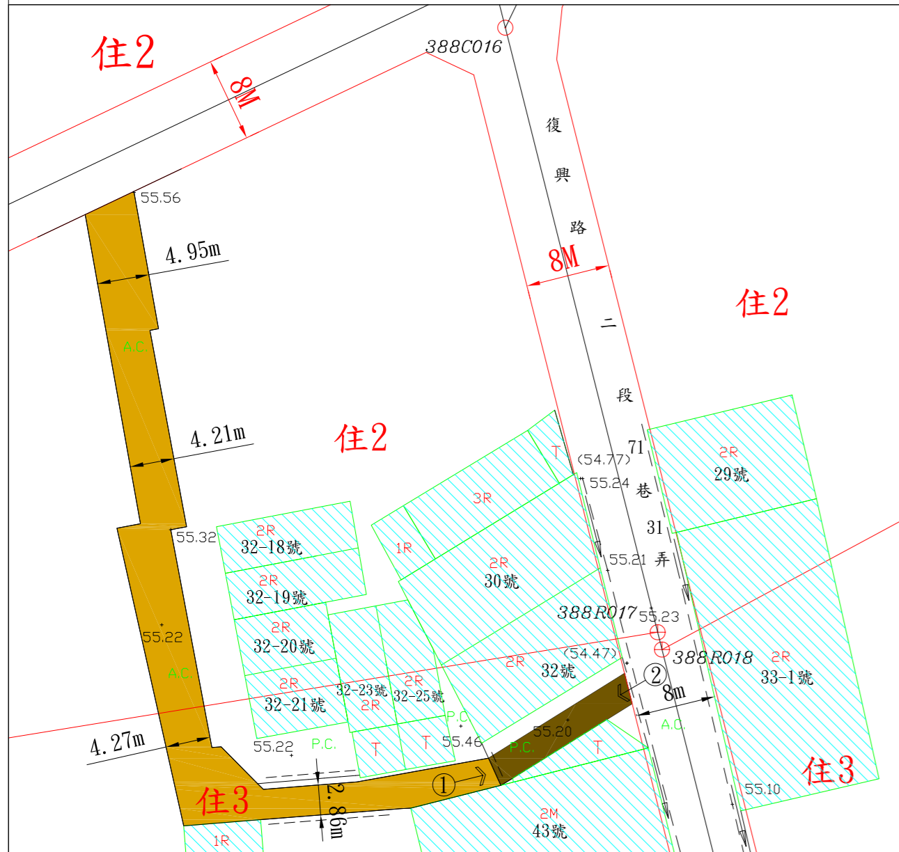
現況圖 SCALE = 1:500
