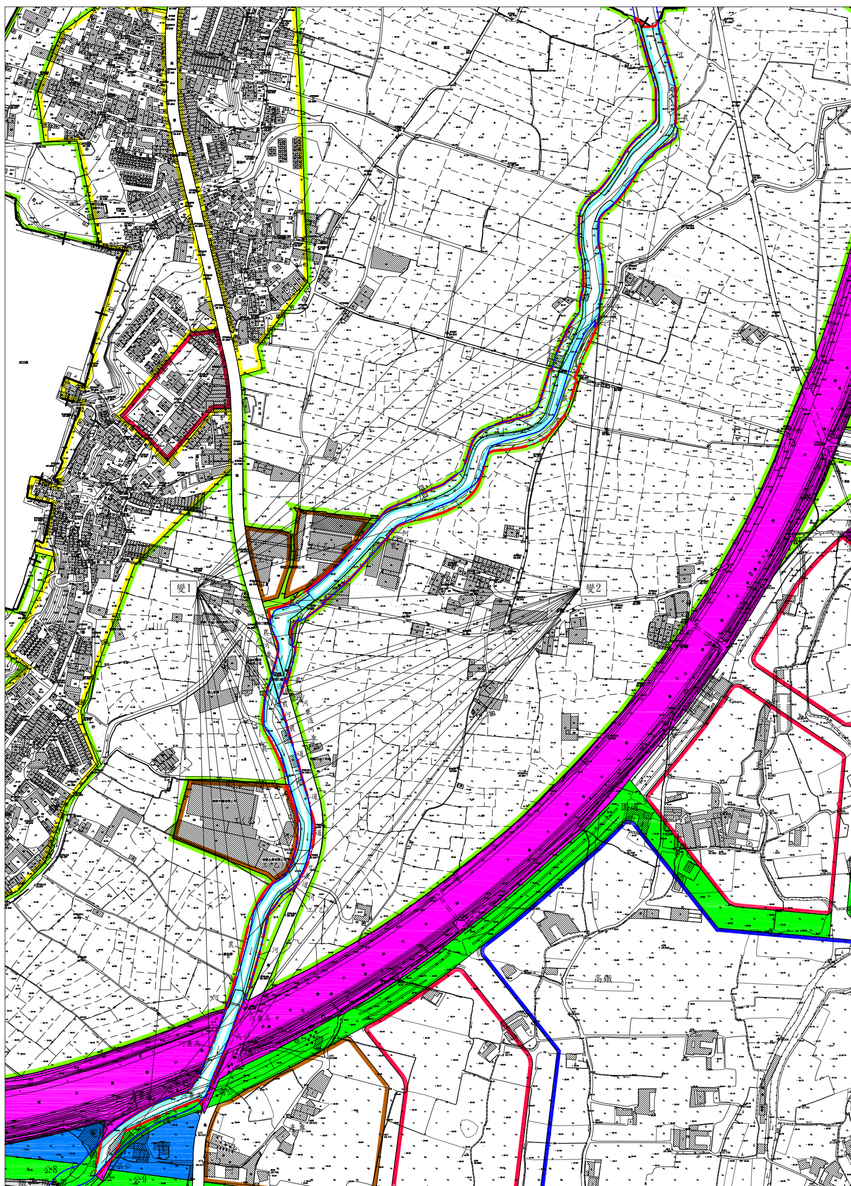
變更臺中市烏日大肚地區都市計畫主要計畫(配合同安厝排水系統一同安厝排水治理計畫(第一次修正))案圖
